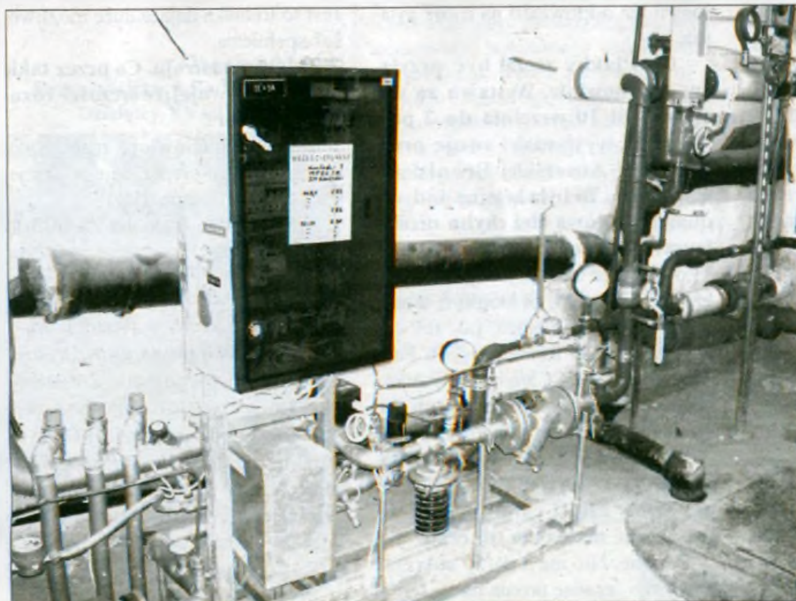
Nowoczesny węzeł cieplny wraz z automatyką pogodową istotnie wpływa na racjonalne zużycie ciepła w budynku.
