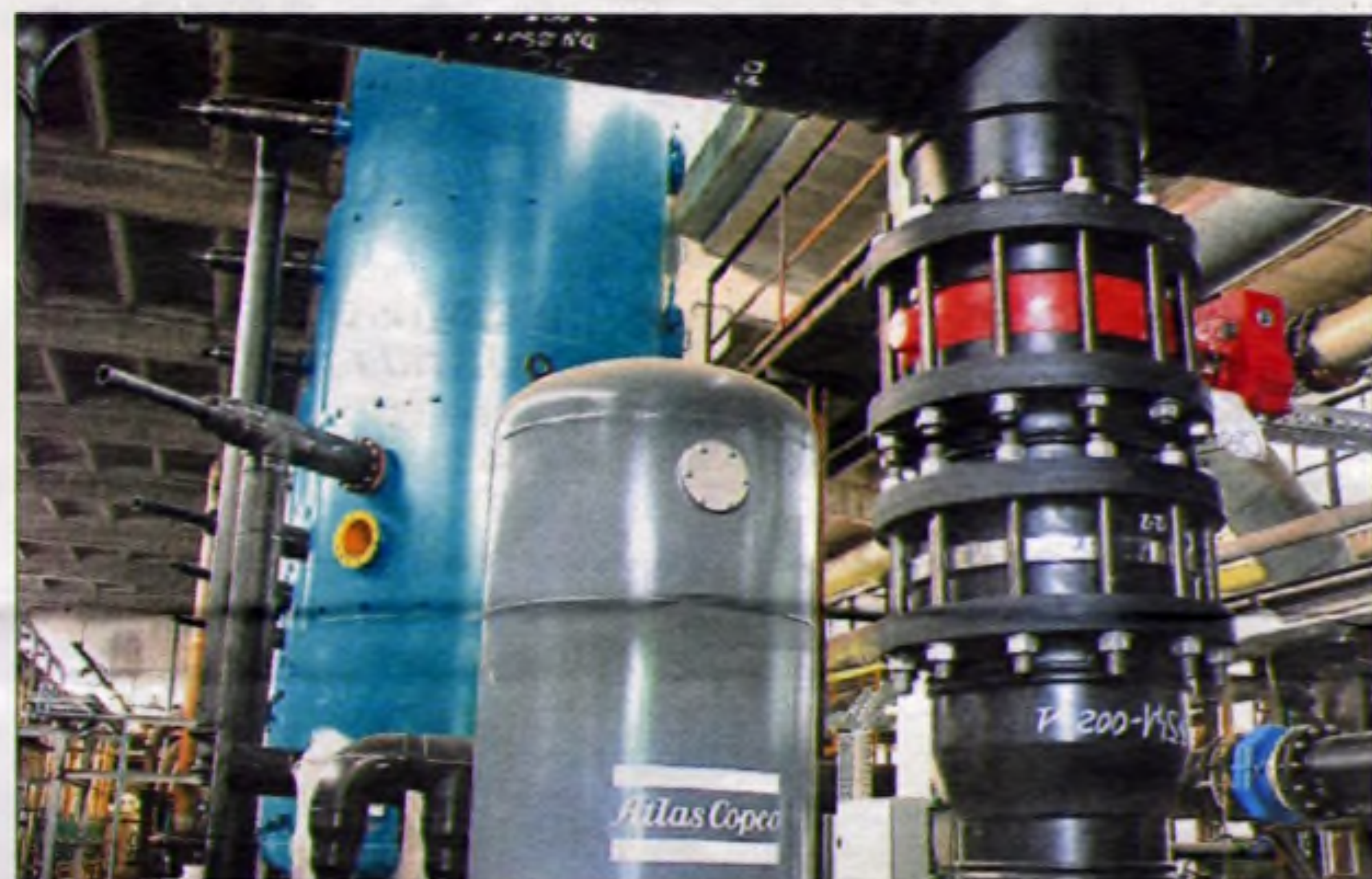
Elementy stacji zmiękczenia w czasie transportu.
